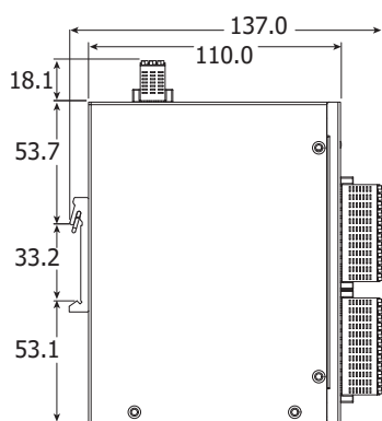
左視圖
