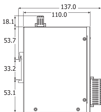
左視圖
